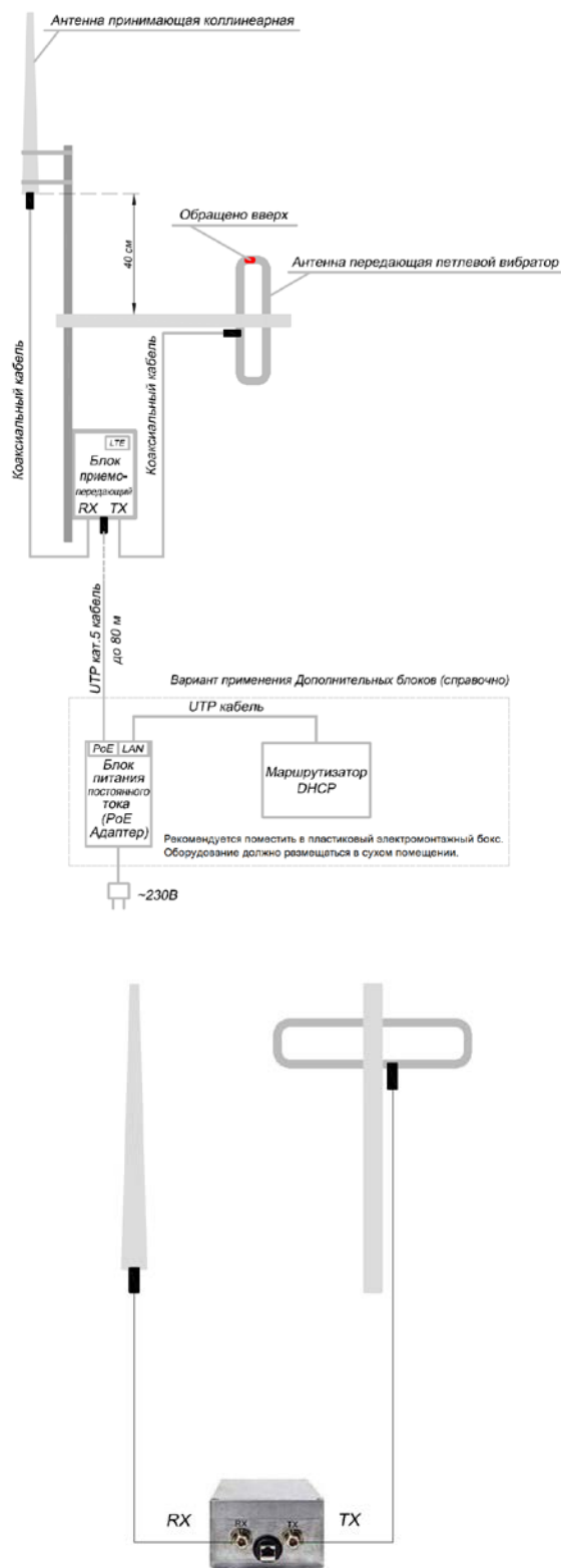
Рисунок А3. Изображения антенно-фидерных устройств, с указанием способа подключения антенн к блоку приемо-передающему Базовой станции NB-Fi
