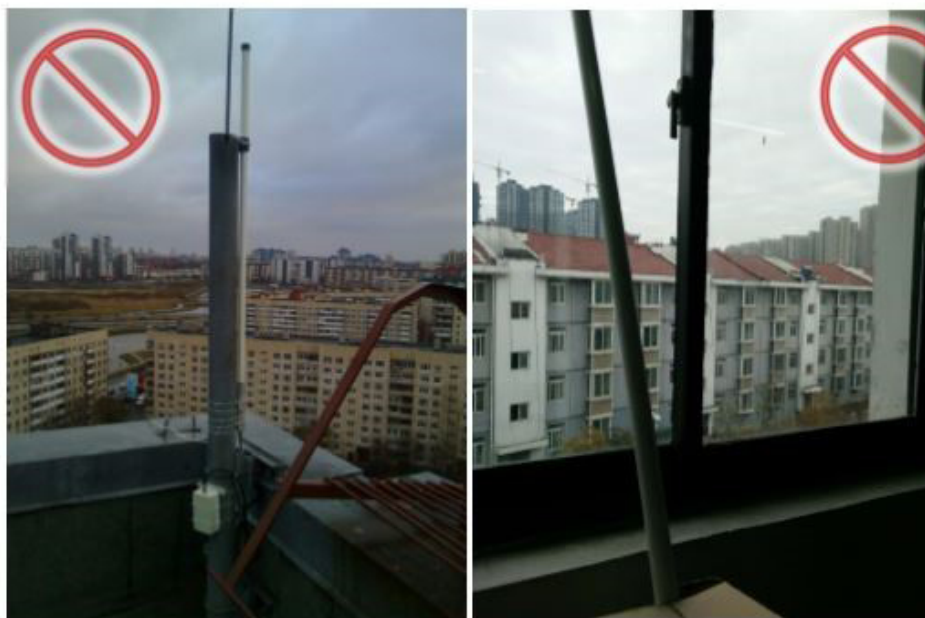
Ошибка! Мачта и молниеотвод закрывают антенну, антенна слишком низко над парапетом (слева); антенна установлена в квартире жилого дома (справа).
